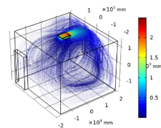
Musterraum mit 48 m 3 Raumvolumen Zirkulation nach 5 min
